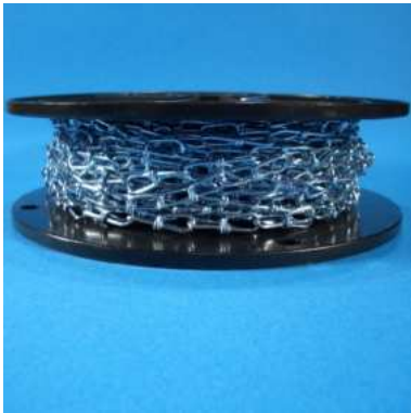
Knotenkette - K16 1,6 mm ø Stahl-verzinkt Innenlänge: 23 mm Außenbreite: 7 mm Art-Nr. 06-106000-01 Verpackungseinheit: 30 m Rolle 15,09 € per Rolle
