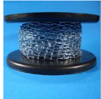
Knotenkette - K14 1,4 mm ø Stahl-verzinkt Innenlänge: 21 mm Außenbreite: 7 mm Art-Nr. 06-104001-01 Verpackungseinheit: 30 m Rolle 14,61 € per Rolle
