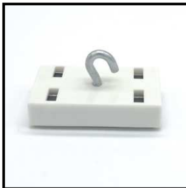
Deckenmagnet weiß, mit Haken kunststoffummantelt Abm.: 53 x 27 x 28 mm Haftkraft: 15 kg Art-Nr. 03-510040-05 Verpackungseinheit: 60 Stück 1,28 € per Stück
