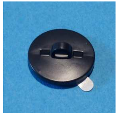
Selbstklebescheibe schwarz mit Öse, rund 20 mm ø Art-Nr. 03-510091-10 Verpackungseinheit: 100 Stück 24,90 € per 100 Stück
