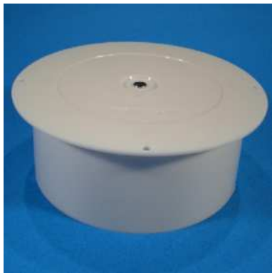
Batteriedrehbühne 4 kg Tragkraft ohne Bodenplatte offener Zugang zum Batteriehalter, weißes Kunststoffgehäu- se, Betrieb mit 1 bzw. 2 Monozellen R20 R1,5V Gehäusedurchmesser: 150 mm Gesamthöhe: 58 mm Drehzahl: 1,7 U/Min. (rechtsdrehend) Art-Nr. 05-035000-08 24,20 € per Stück
