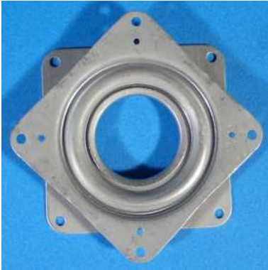
Kugellager 75 x 75 x 8 mm aus verzinktem Stahlblech Innen- \varnothing : 33 mm max. Auflage: bis 45 cm \varnothing max. Belastung: 90 kg Art-Nr. 05-075075-04 3,95 € per Stück
