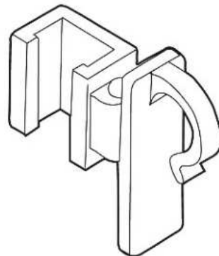
Aufhängehaken 2-teilig zum einhängen von Rahmen an Drahtgittern bis max. 12 mm \varnothing , grau Art-Nr. 08-100136-15 Verpackungseinheit: 10 Paar 1,16 € per Paar
