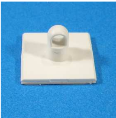
Rotating Clip , weiß, drehbar selbstklebend, 30 mm x 30 mm Art-Nr. 15-252700-05 Verpackungseinheit: 100 Stück 18,90 € per 100 Stück
