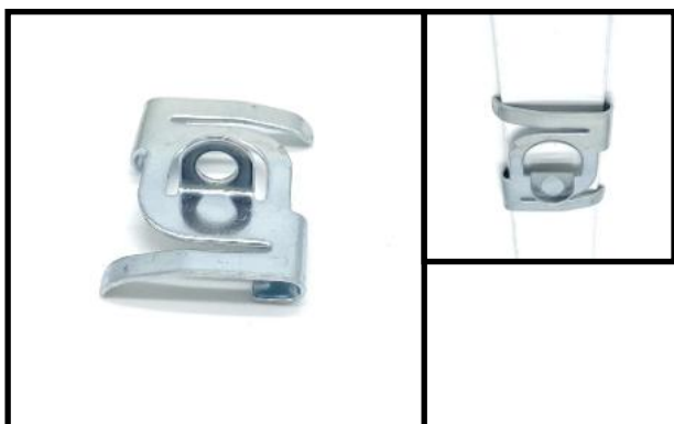
Decken-Clip , verzinkt 38 x 28 mm, Öse: 5 mm \varnothing Art-Nr. 01-118000-01 Verpackungseinheit: 100 Stück 99,00 € per 100 Stück
