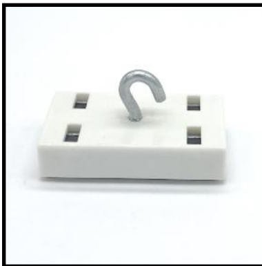
Deckenmagnet weiß, mit Haken kunststoffummantelt Abm.: 53 x 27 x 28 mm Haftkraft: 15 kg Art-Nr. 03-510040-05 Verpackungseinheit: 60 Stück 1,34 € per Stück
