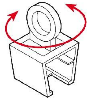
Aufhängeöse drehbar mit Öse zum Aufhängen, stufenlos drehbar, transparent Art-Nr. 08-102101-00 Verpackungseinheit: 100 Stück Preis: auf Anfrage
