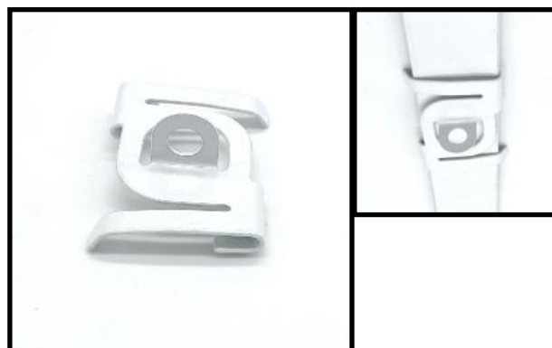
Decken-Clip , weiß 38 x 28 mm, Öse: 5 mm \varnothing Art-Nr. 01-118000-05 Verpackungseinheit: 100 Stück 105,00 € per 100 Stück
